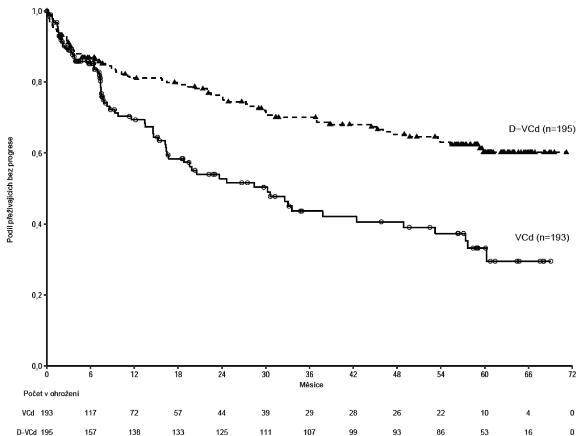
Obrázek 4: Kaplanova-Meierova křivka MOD-PFS ve studii AMY3001
