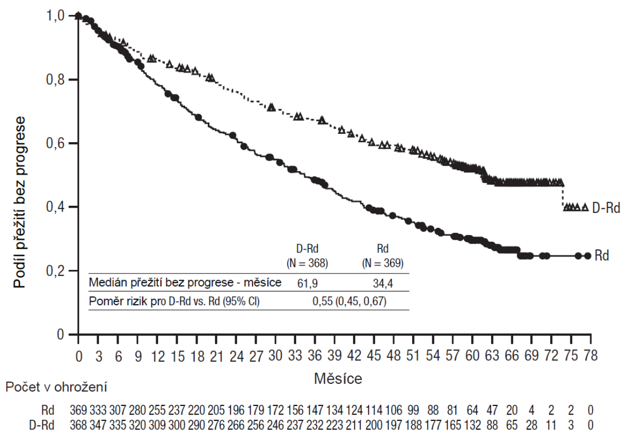
Obrázek 6: Kaplanova-Meierova křivka PFS ve studii MMY3008
