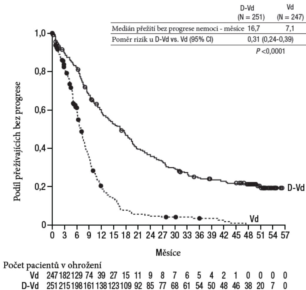
Obrázek 13: Kaplanova-Meierova křivka PFS ve studii MMY3004
