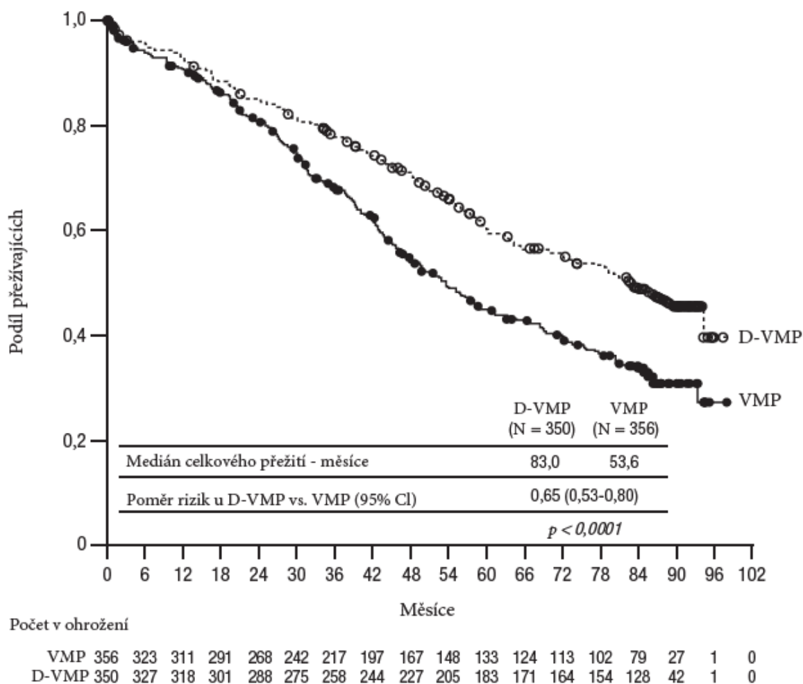
Obrázek 9: Kaplanova-Meierova křivka OS ve studii MMY3007
