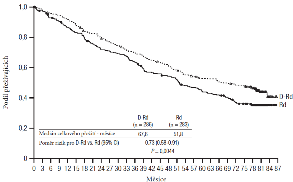
Obrázek 12: Kaplanova-Meierova křivka OS ve studii MMY3003
