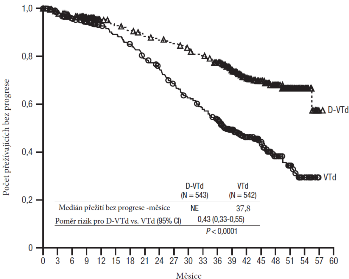
Obrázek 10: Kaplanova-Meierova křivka PFS ve Studii MMY3006
