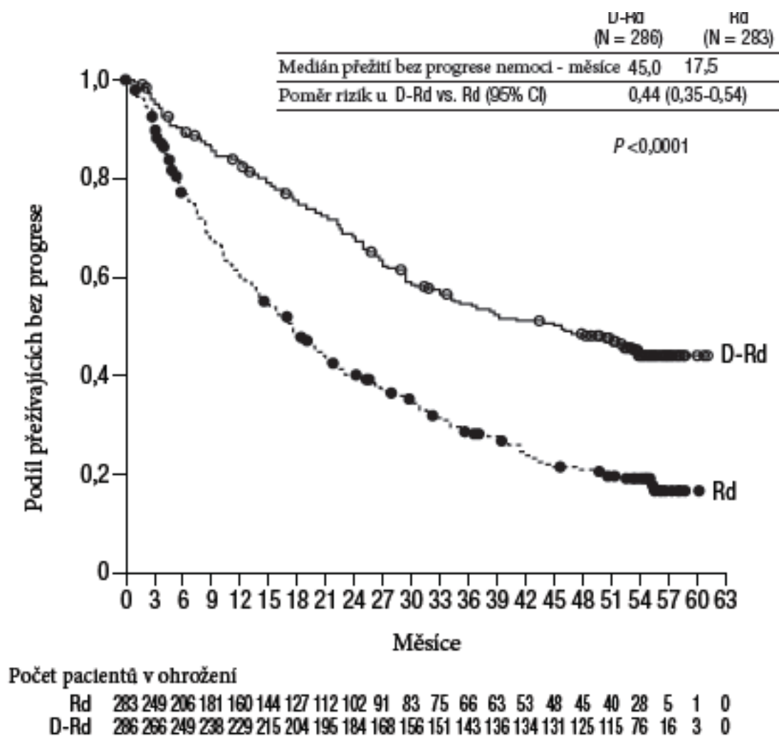
Obrázek 11: Kaplanova-Meierova křivka PFS ve studii MMY3003
