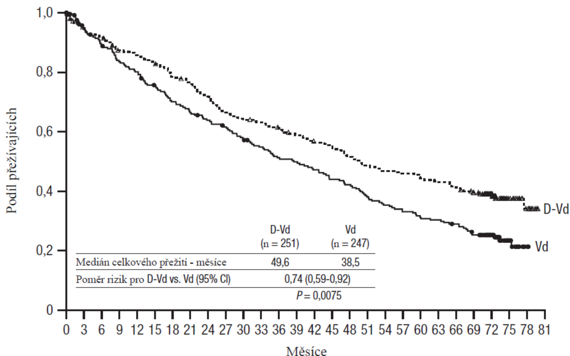
Obrázek 14: Kaplanova-Meierova křivka OS ve studii MMY3004
