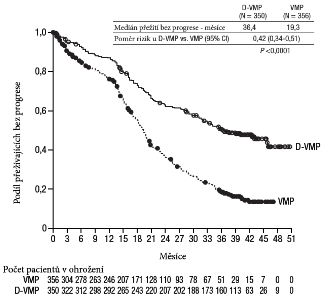
Obrázek 8: Kaplanova-Meierova křivka PFS ve studii MMY3007
