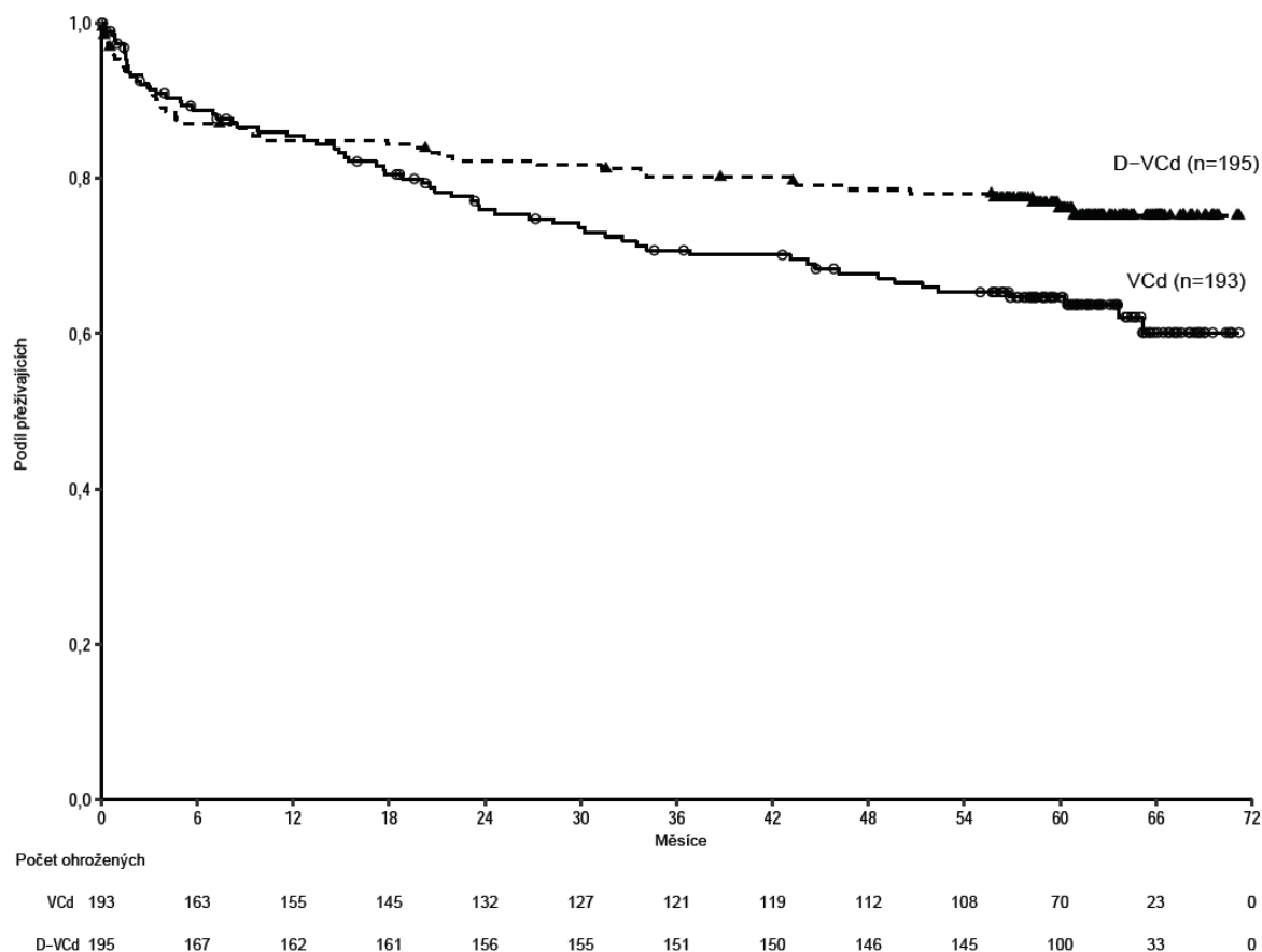
Obrázek 5: Kaplanova-Meierova křivka OS ve studii AMY3001
