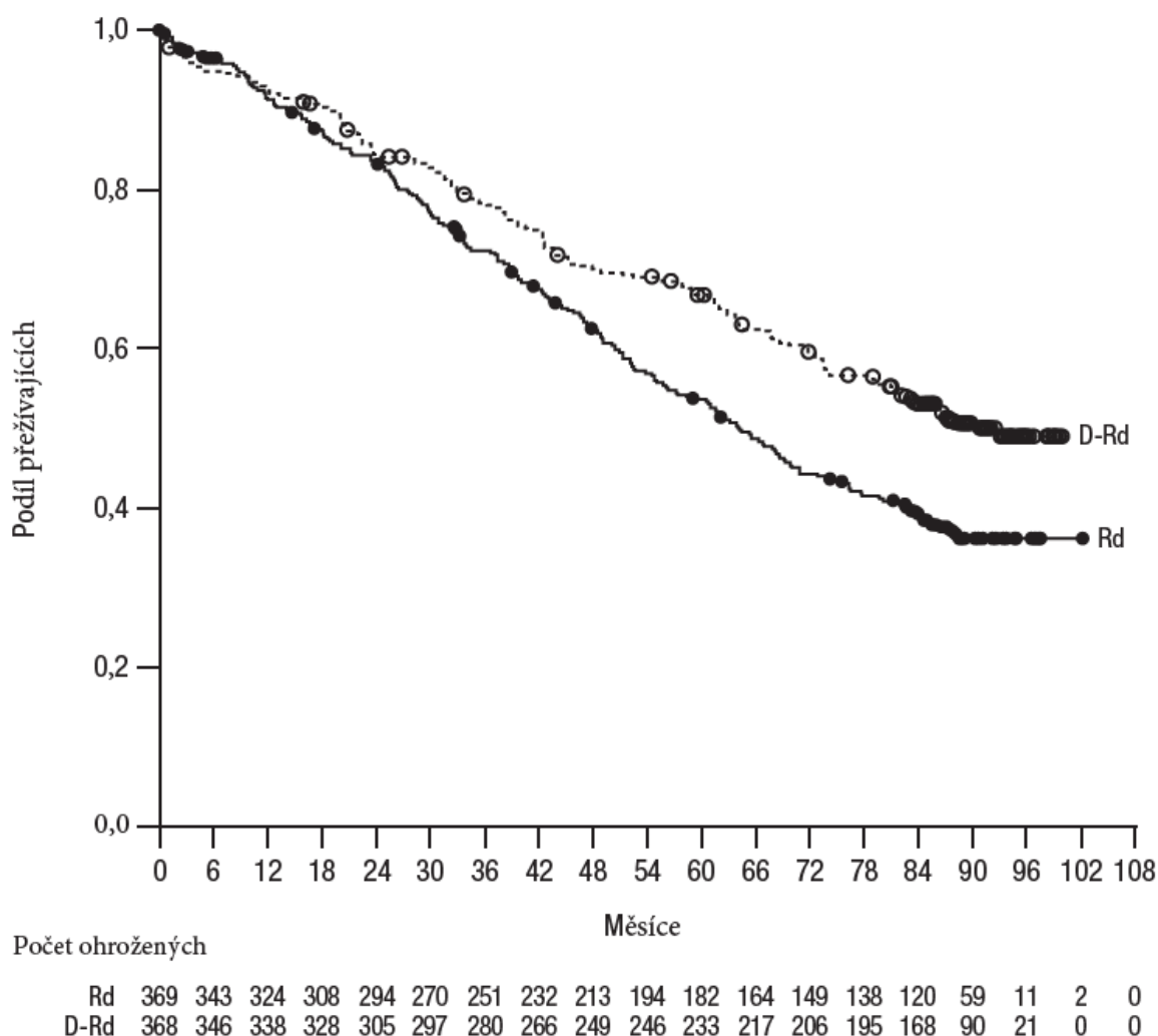
Obrázek 7: Kaplanova-Meierova křivka OS ve studii MMY3008
